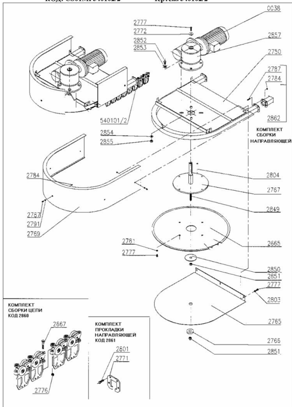
СХЕМА 2/2. БЛОК ПРИВОДА 1,1 кВт – для многоуровневых конвейеров и одноуровневых конвейеров протяженностью более 500 ячеек КОД: CS01MP540102/2 Чертеж. 540102/2
