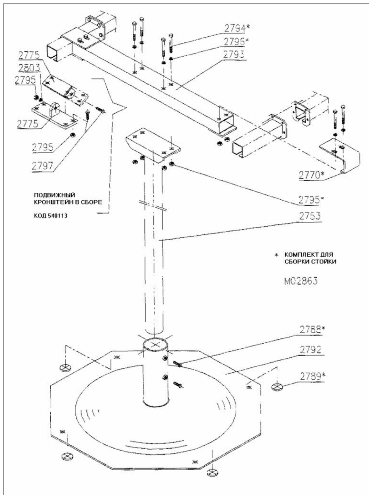
СХЕМА 3. ОПОРНАЯ СТОЙКА КОД: CS10TS540112P (1-2-3)
