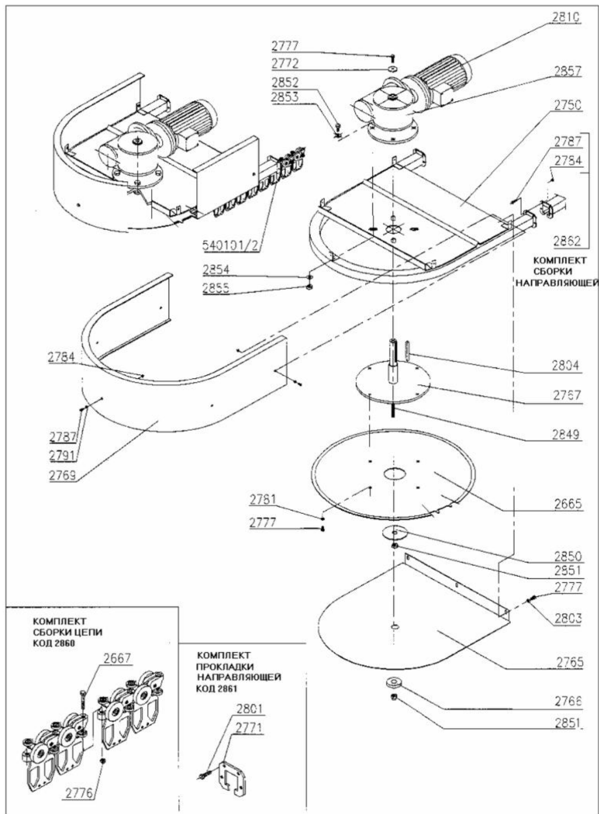
СХЕМА 2/1. БЛОК ПРИВОДА 1,5 кВт – для многоуровневых конвейеров КОД: CS01MP540102/1 Чертеж. 540102/1
